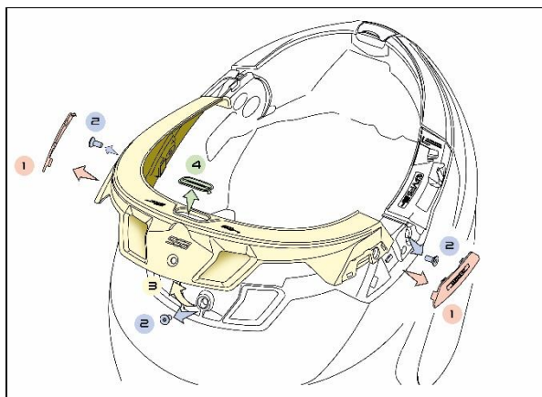
Obr. 4C - POUZE PRO PŘÍLBY N100-6, N120-1
