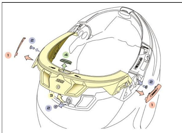
SI. 4C – SAMO ZA ČELADE N100-6, N120-1
